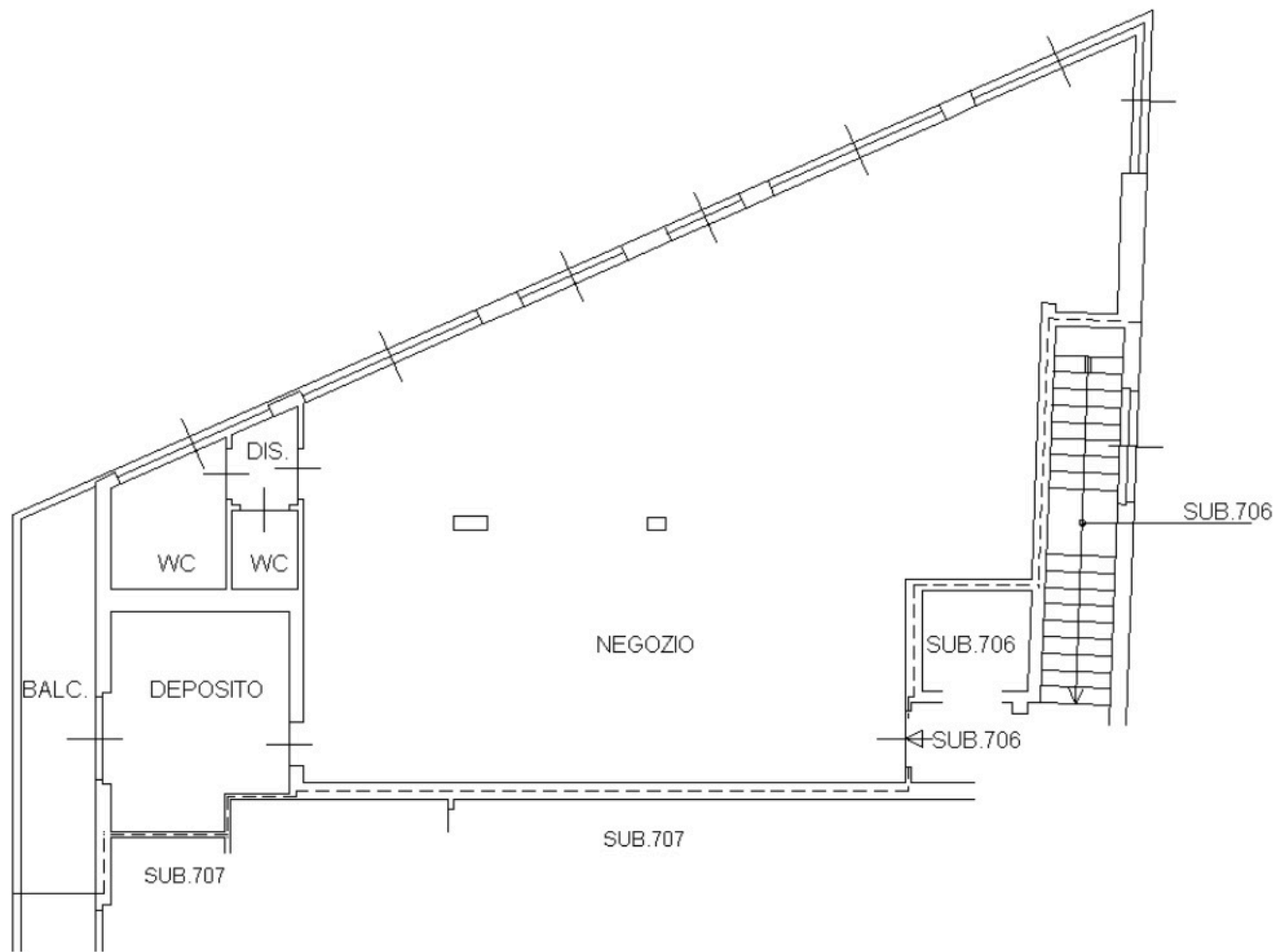
PIANTA PIANO PRIMO H=2.95 MT
